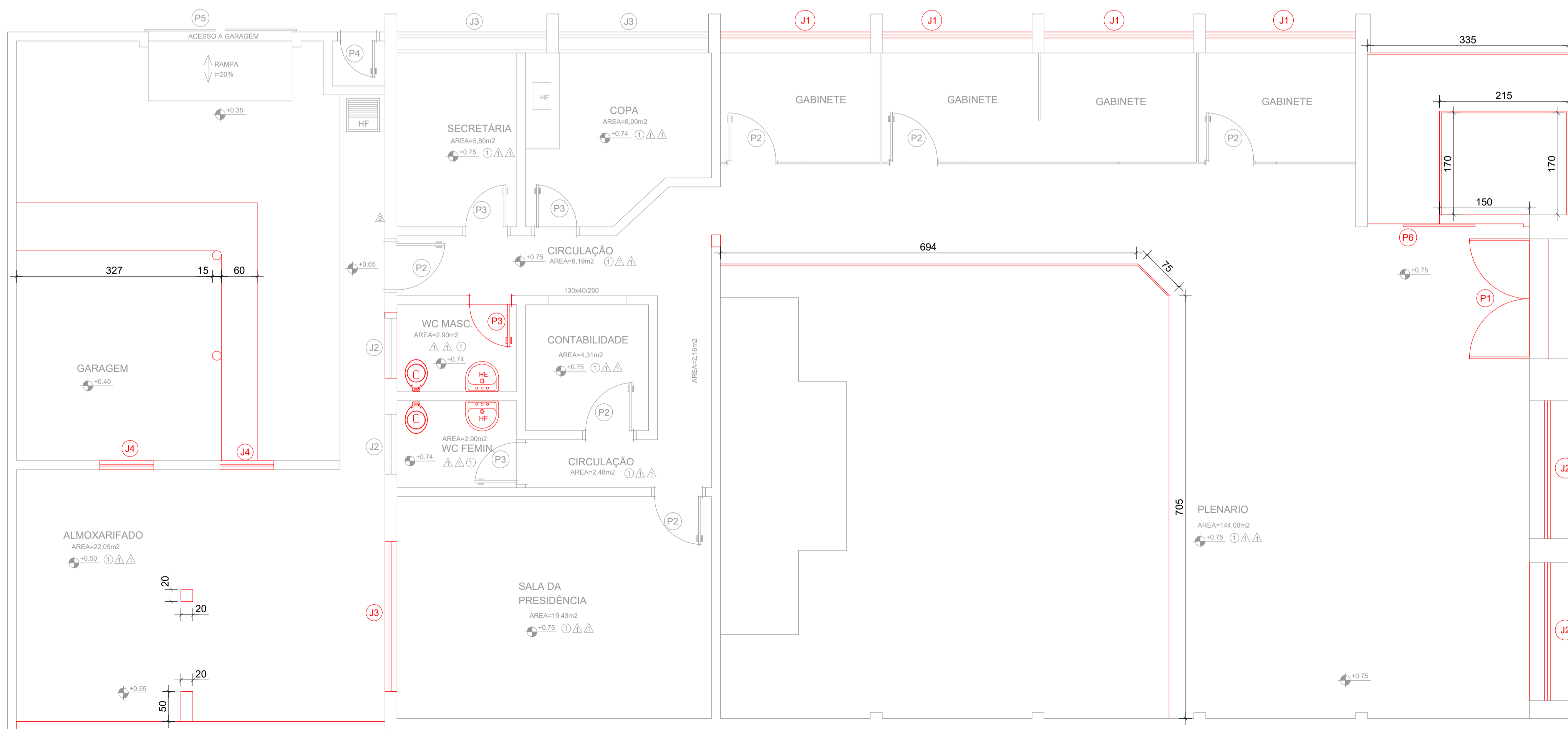
PLANTA BAIXA DEMOLIÇÃO ESC. 1:50
